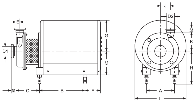
SFB-70外形安装尺寸 Dimensions
