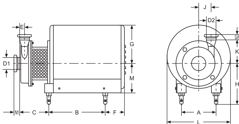
SFB-10外形安装尺寸 Dimensions
