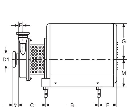
SFB-15外形安装尺寸 Dimensions
