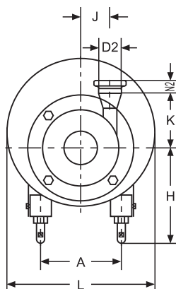
SFB-15外形安装尺寸 Dimensions
