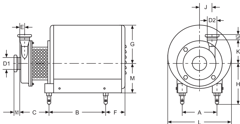
SFB-20外形安装尺寸 Dimensions
