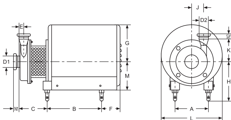
SFB-5外形安装尺寸 Dimensions
