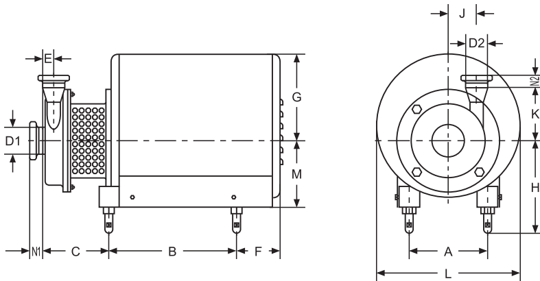
SFB-40外形安装尺寸 Dimensions
